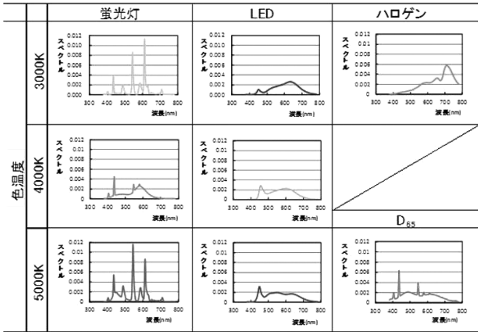
図2 各光源の分光分布図
